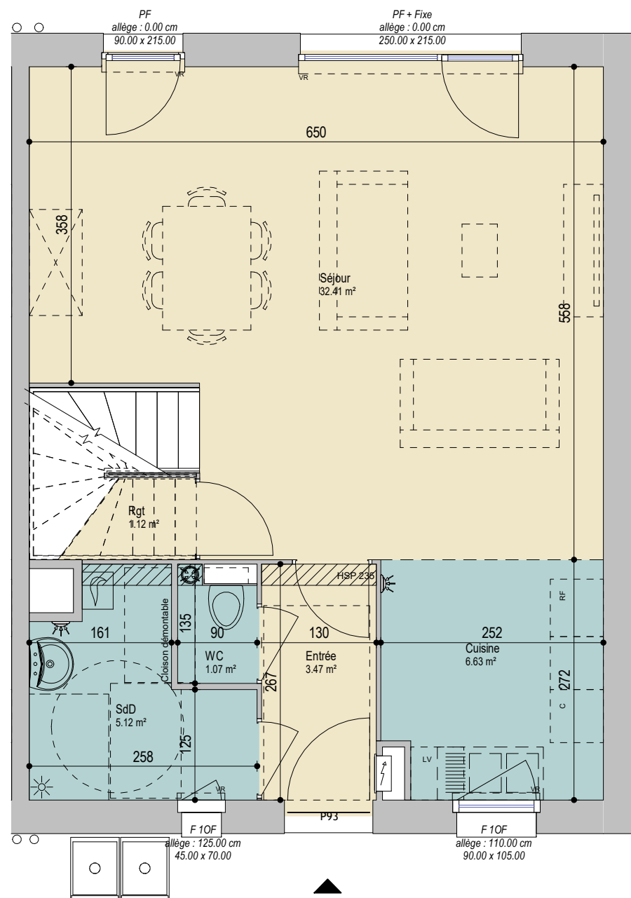
Maison 10
