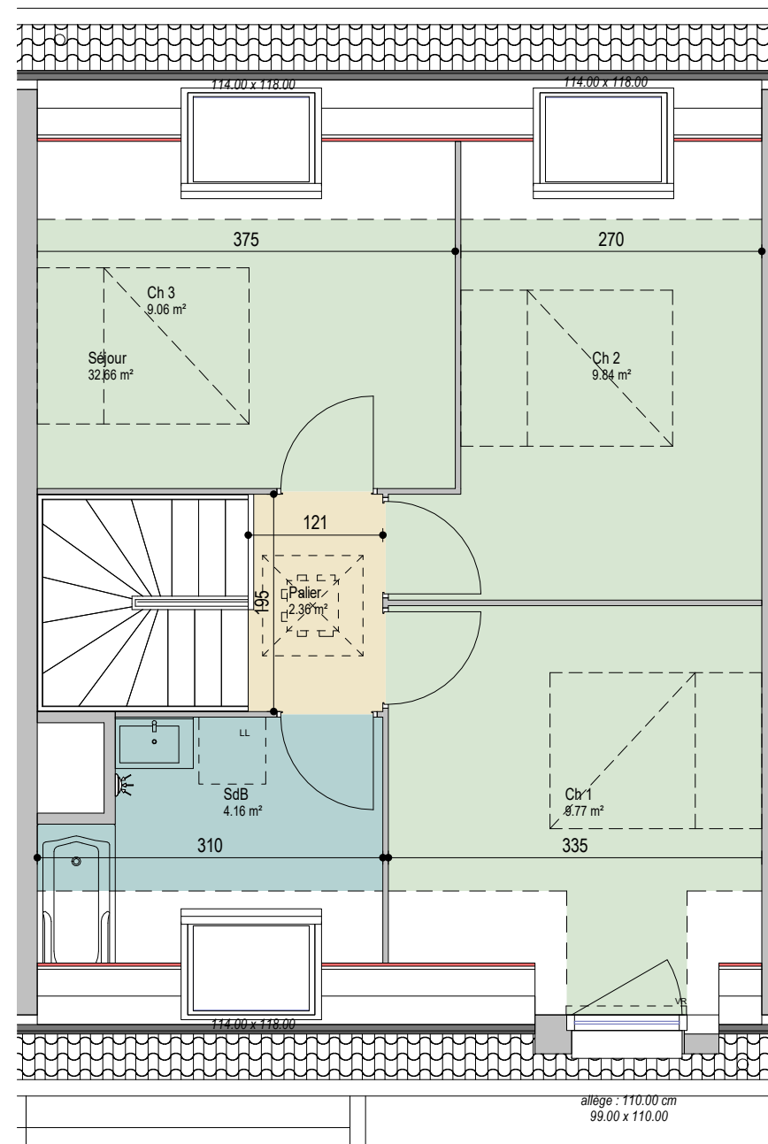
2 Etage Ech : 1 : 60
