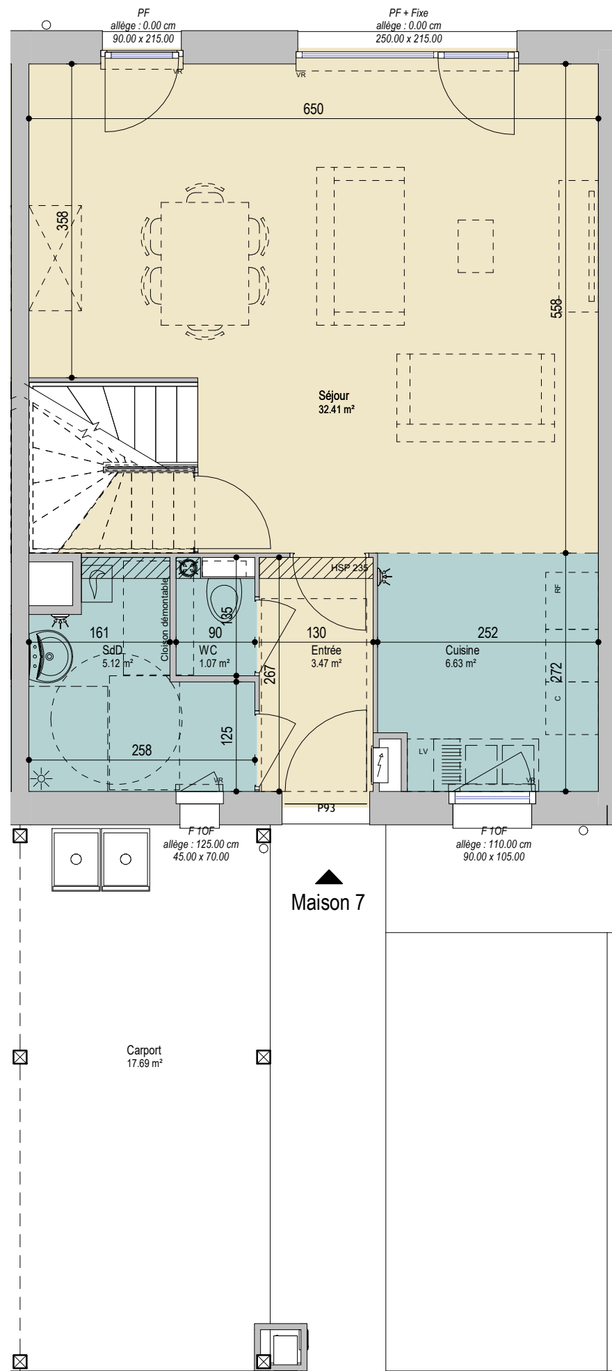
1 Rez-de-chaussée Ech : 1 : 60
