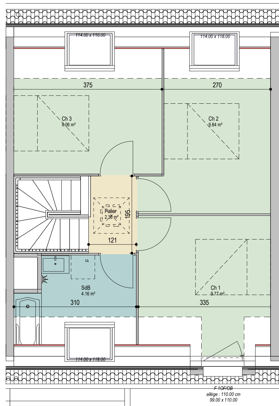
1 Etage Ech : 1 : 60
