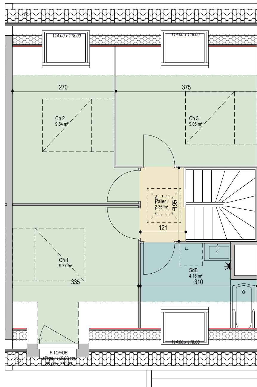
2 Etage Ech : 1 : 60
