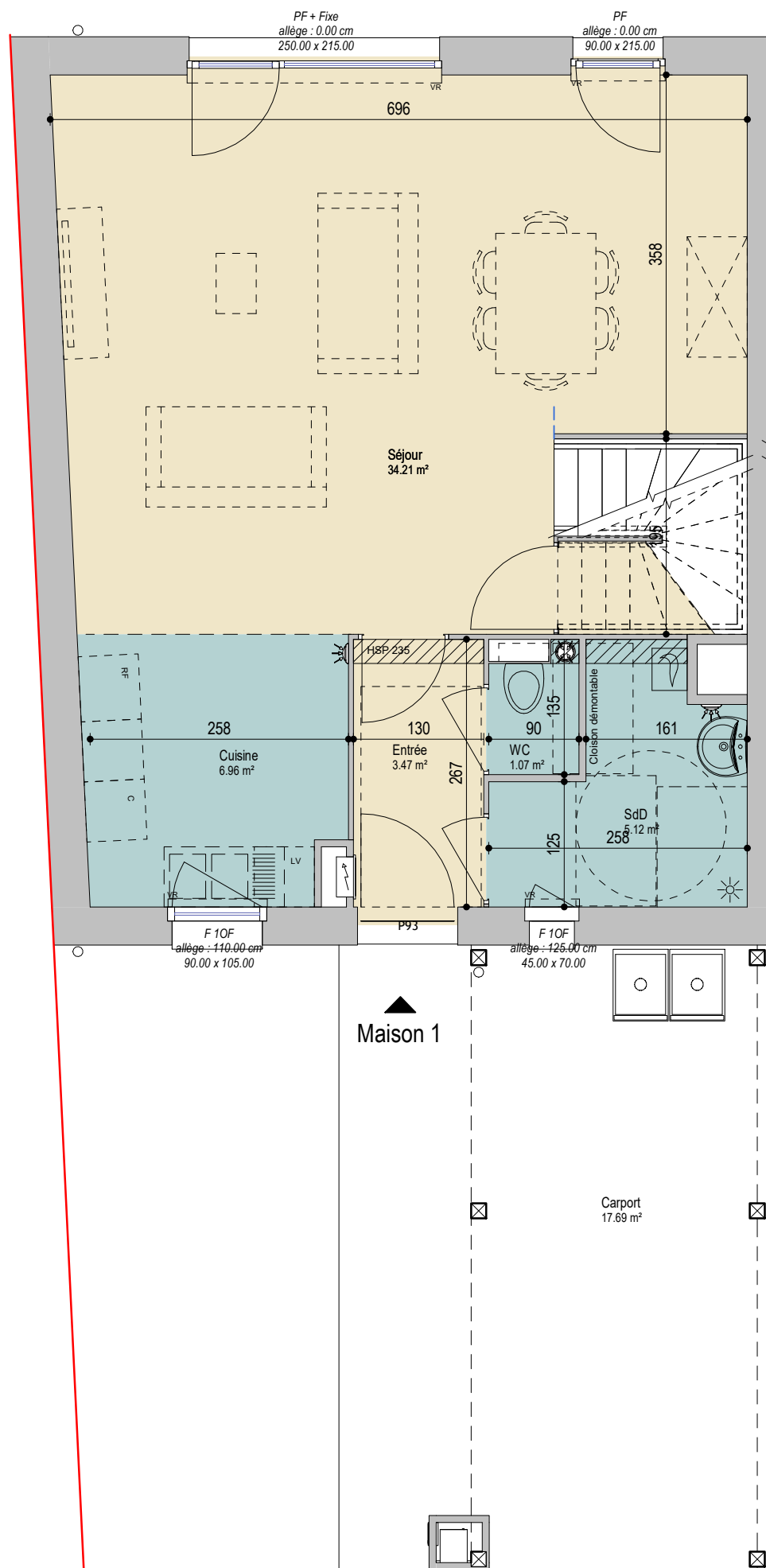
1 Rez-de-chaussée Ech : 1 : 60
