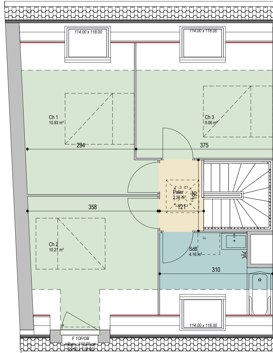
2 Etage Ech : 1 : 60
