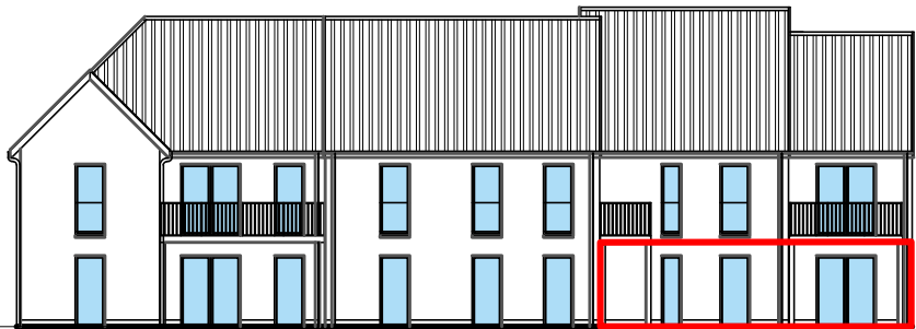
façade OUEST
