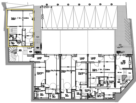
Plan rez-de-chausée
