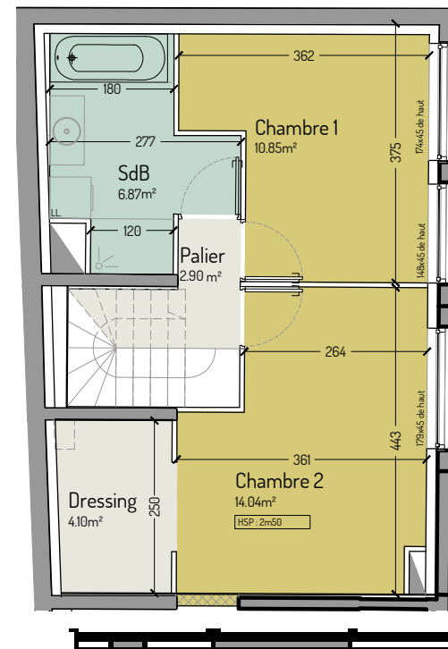
Plan entresol
