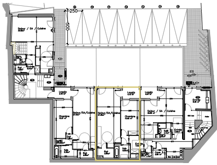
Plan rez-de-chaussée
