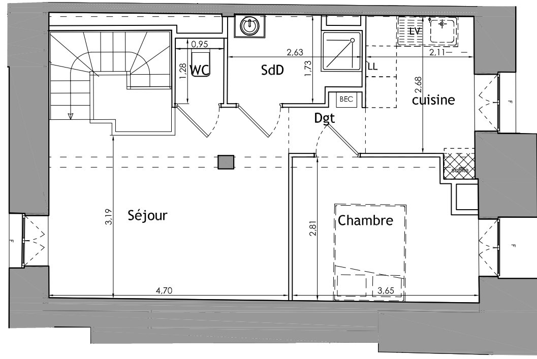
Entresol (hauteur sous plafond ≈ 2,15m)
