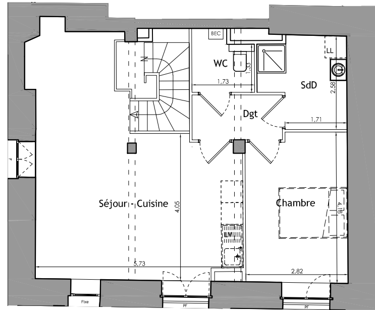
Entresol (hauteur sous plafond ≈ 2,15m)
