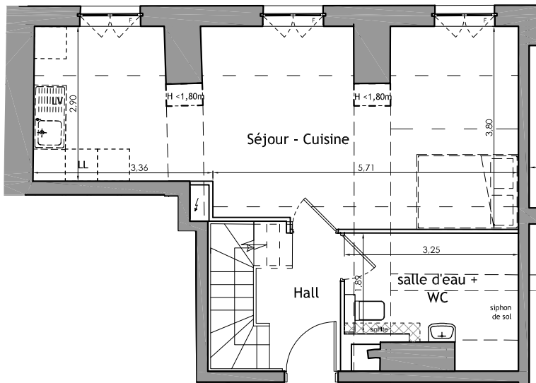
R+3 (hauteur sous plafond ≈ 2,20m)
