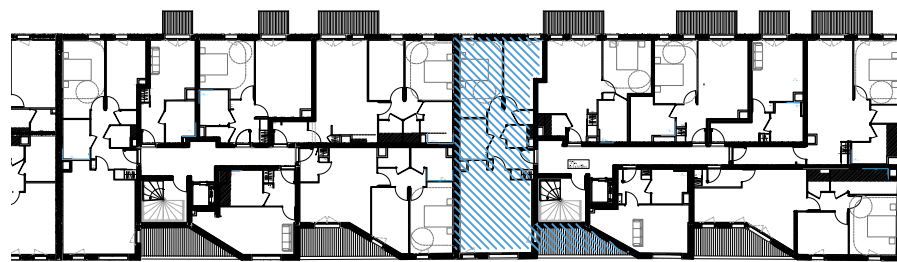
Repérage - Plan R+2
