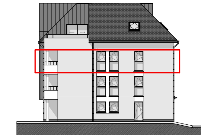
Façade Est
