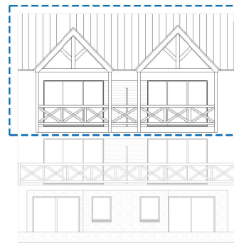
Façade Ouest
